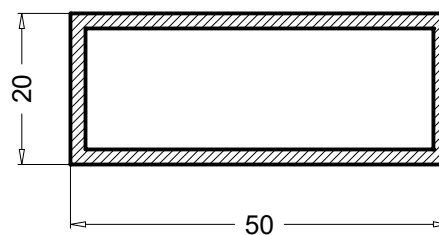
TR50202 0.712 Kg/m
