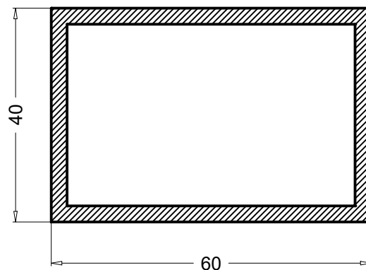
TR60403 1.522 Kg/m
