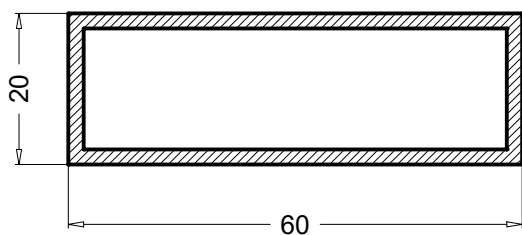
TR60202 0.820 Kg/m
