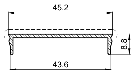
PM14004 0.244 Kg/m
